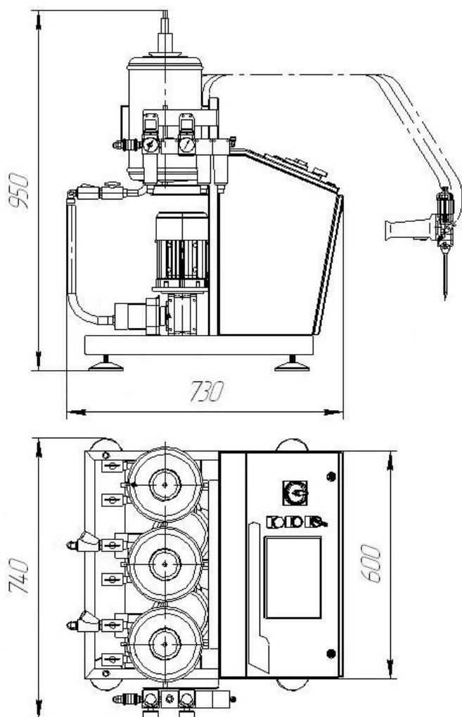
Дозирующая машина Компакт 2.
