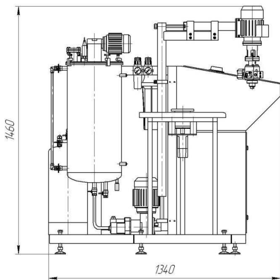
Дозирующая машина LP2-02 – исполнение с рабочим столом с поворотным устройством с сервоприводом.
