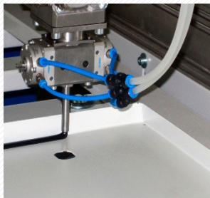
Координатный манипулятор ВЕКТОР МЭУ
